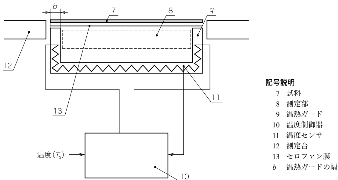
図 A.2—測定部及び温度制御付き温熱ガードの概要
